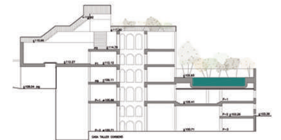
SECCIÓ
