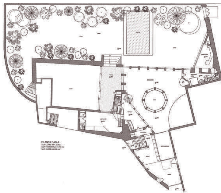
PLANTA BAIXA
